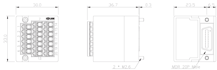
■ 外観図
