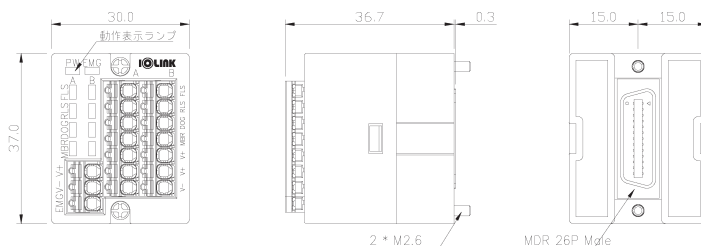
■ 外観図
