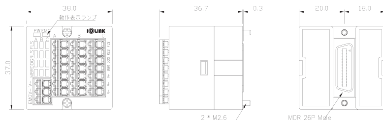
■ 外観図
